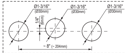
SIZE AND SPACING OF ASSEMBLY OPENINGS TAMAÑOS Y DISTRIBUCIÓN DE LOS ORIFICIOS DE MONTAJE
